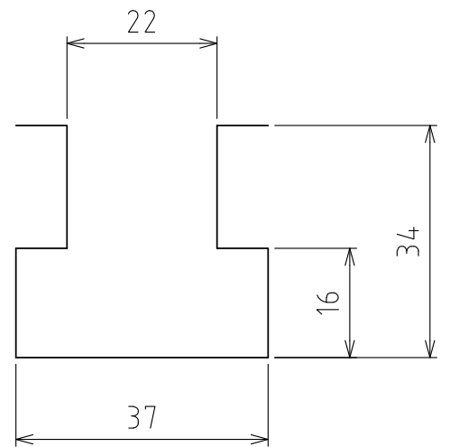
T形槽尺寸
