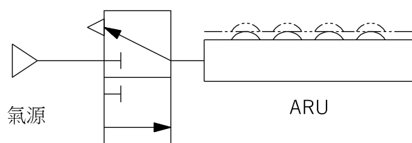
二位三通閥
